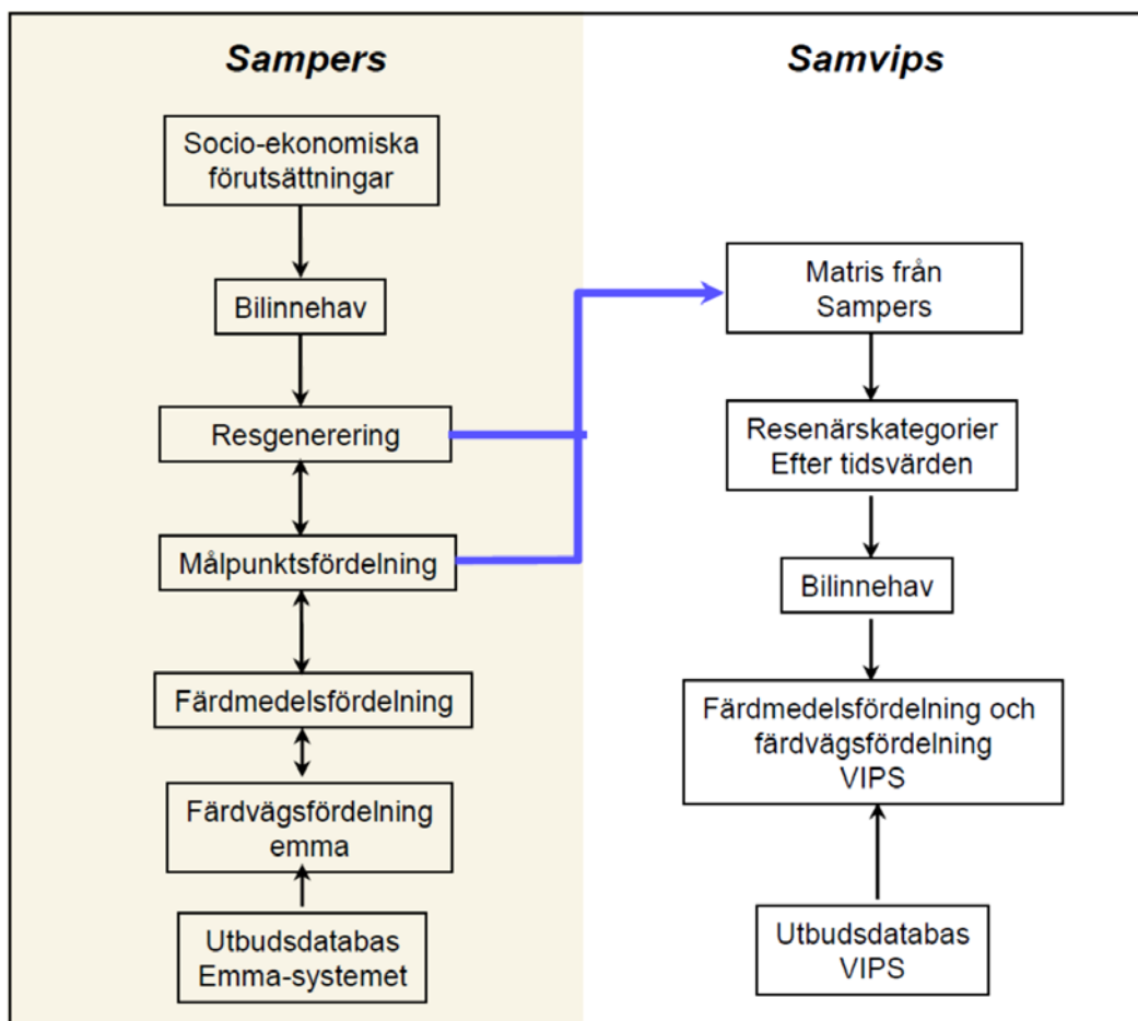
Figur 6: Sammenheng mellom Sampers og Samvips prognosesystem (Nelldal, Jansson og Halldin, 2009)
